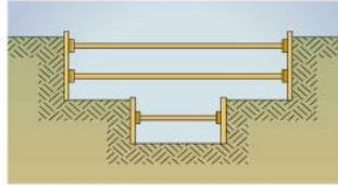
Figura 7 - Escavação tabulada (escavação com paredes em tabuleis)
