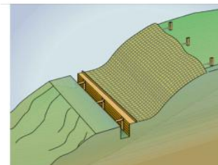
Figura 9 - Escavação aberta - com paredes em taludes e com paredes protegidas por cortinas
