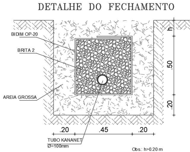
Figura 9 - Detalhe de trincheira drenante.
